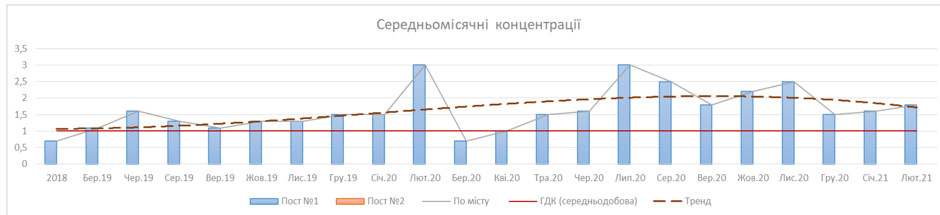
Рисунок 6.15. Графік середньомісячних концентрацій формальдегіду
