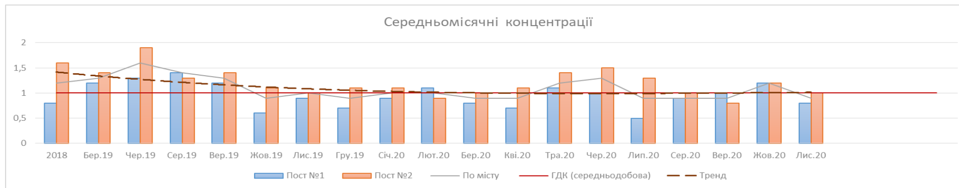
Рисунок 6.17. Графік середньомісячних концентрацій фтористого водню
