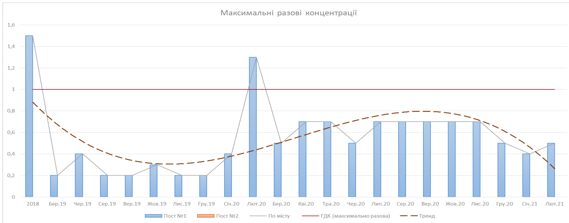
Рисунок 6.14. Графік максимальних разових концентрацій формальдегіду
