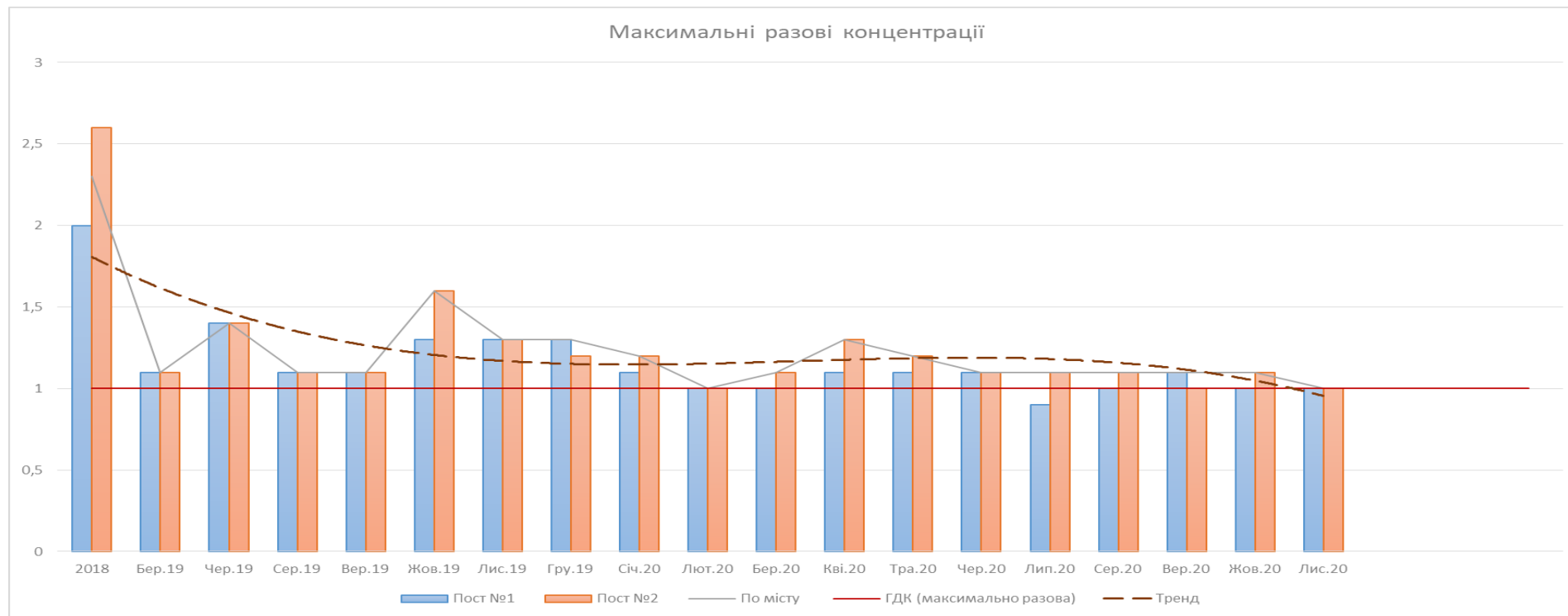
Рисунок 6.16. Графік максимальних разових концентрацій фтористого водню
